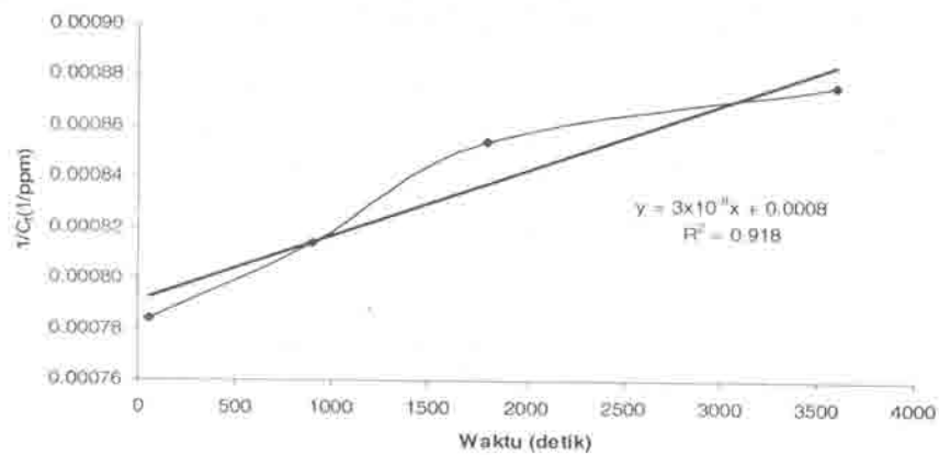
Gambar 6. Grafik 1/C_t lawan t untuk reaksi pertukaran anion sulfat oleh Cr_2O_7^{2-}
