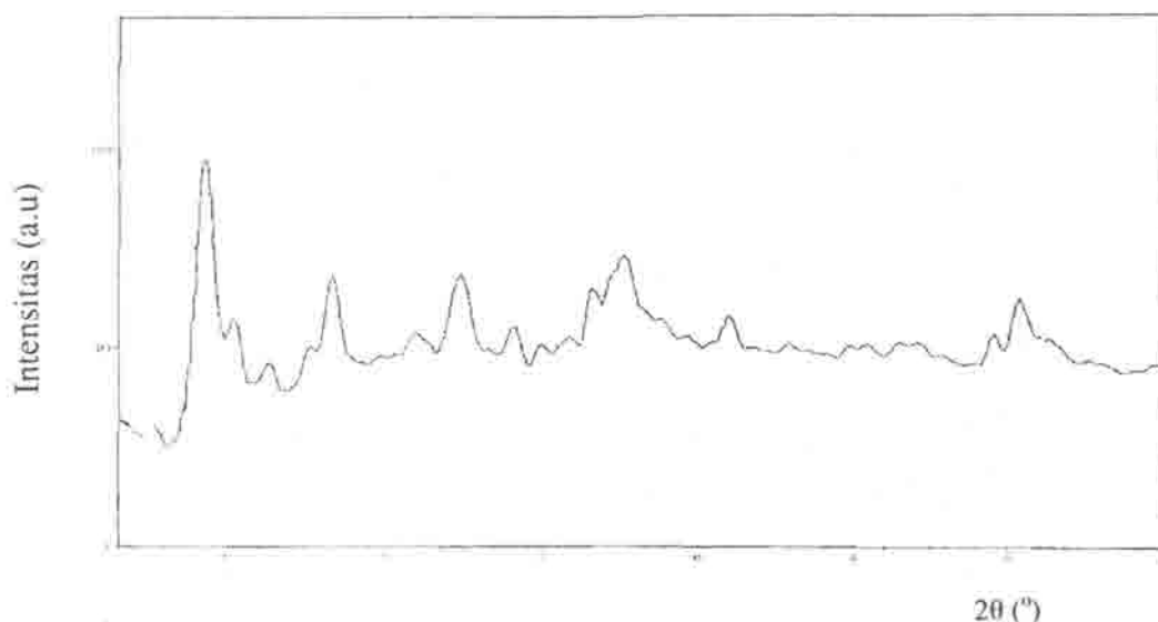
Gambar 2. Difraktogram hidrotalsit Zn-Al-SO_4 hasil sintesis
